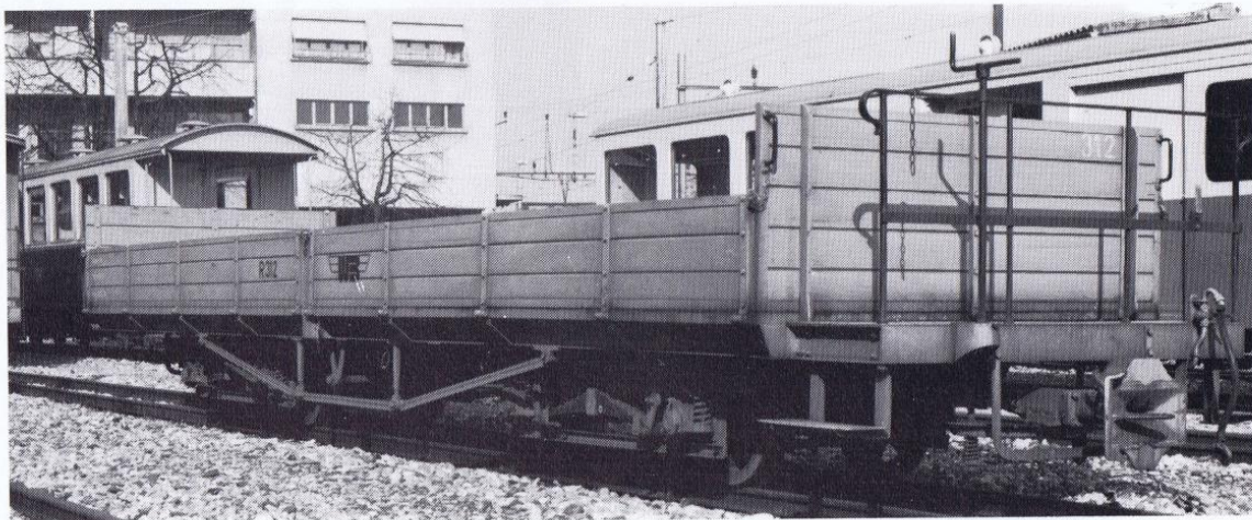
Vierachsiger Flachwagen R 312, 1957 mit Teilen des BC 4 13 gebaut
